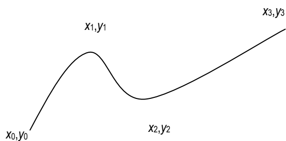
Рис. 1. Кривая Безье
